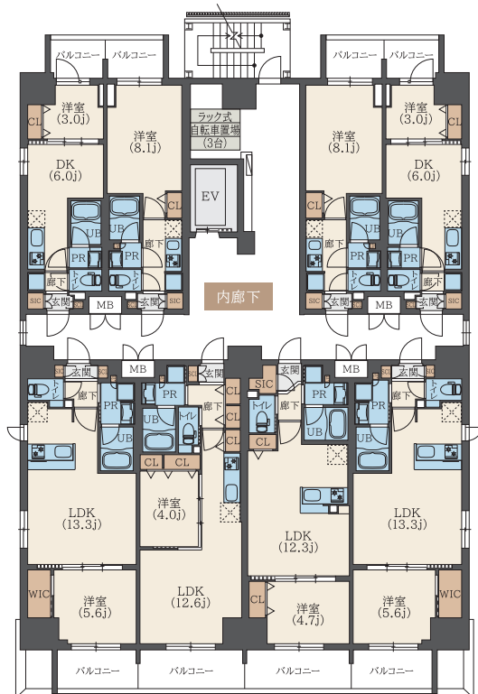
3F~10F平面図
